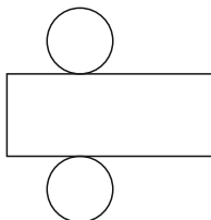
Zylinder
