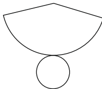
Kegel
